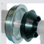
GAR113 (Ø 118-174mm) Furgoni Vans and light trucks Lieferwagen und LLKW's Fourgons et petits camions Furgonetas
