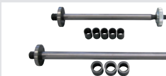
GAR 182 (Ø 12 mm) Albero completo di 1 ghiera e 5 bussole. Shaft including 1 ring nut and 5 bushes. Welle komplett mit Spannvorrichtung und 5 Hülsen. Arbre équipé d'une bague de serrage et 5 manchons. Eje completo de 1 garra y 5 casquillos.
