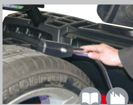
• измерение эксцентricности колеса
