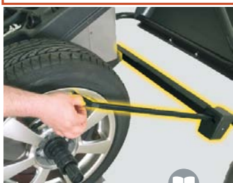
GAR 213 GAR 213 B Устройство автоматического ввода ширины колеса
